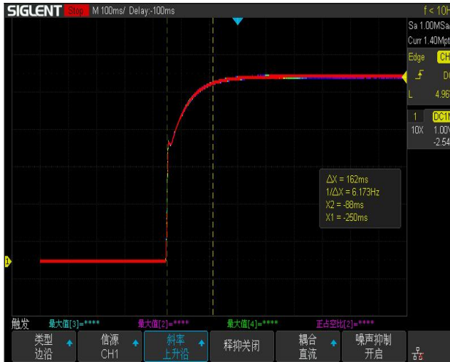
图(5) 25%~50%负载动态波形
