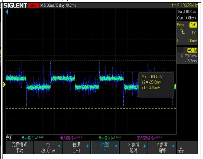
图(6) 50%~75%负载动态波形
