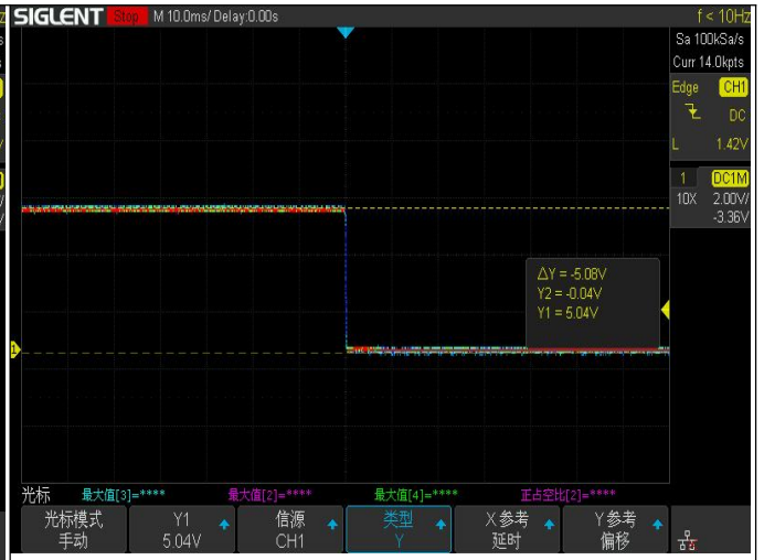
图(6) 50%~75%负载动态波形
